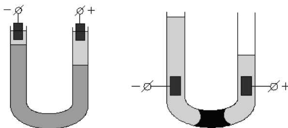
Рис. 6. Схема опыта по электрофорезу и по электроосмосу
