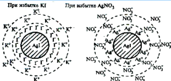
Рис. 3. Строение коллоидных частиц иодида серебра(I)
