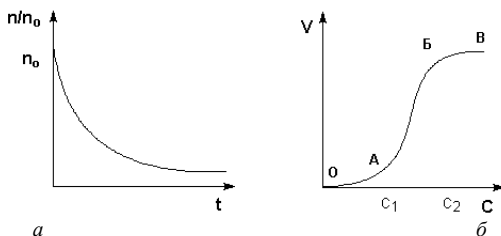
Рис. 7. Коагуляционная кривая (а) и зависимость скорости коагуляции от концентрации (б)
