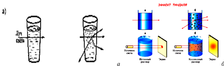
Рис. 4. Эффект светорассеяния при прохождении луча света через коллоидный раствор:
