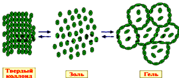
Рис. 1. Строение геля и золя
